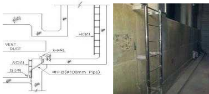
그림 22. 일반사다리 설계 예
