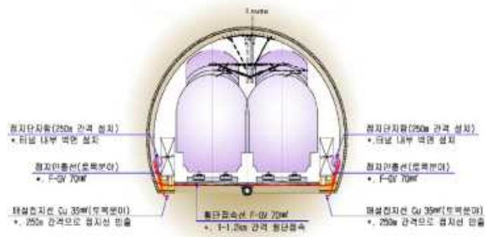
그림 37. 터널구간 접지설계 예(복선)
