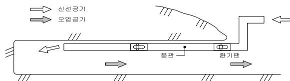
그림 45. 직렬 급기식 환기개요도
