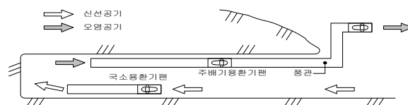
그림 42. 직렬 배기식(덕트 내 부압)
