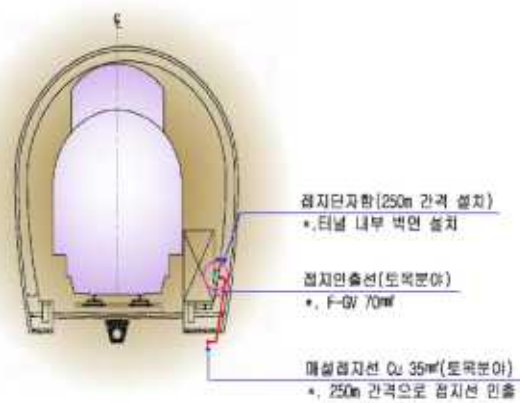
그림 38. 터널구간 접지설계 예(단선)
