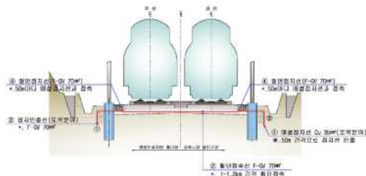
그림 28. 깎기구간 접지설계 예
