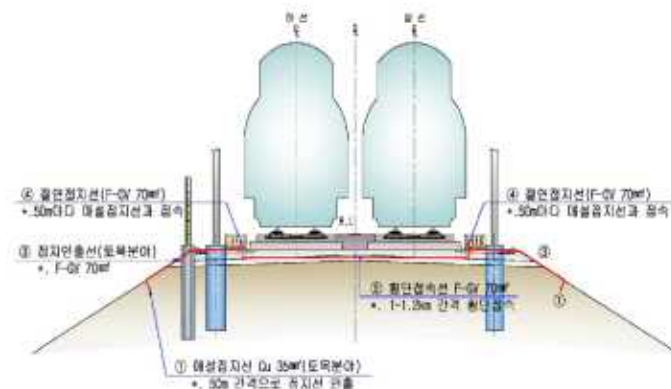
그림 27. 흙쌓기구간 접지설계 예
