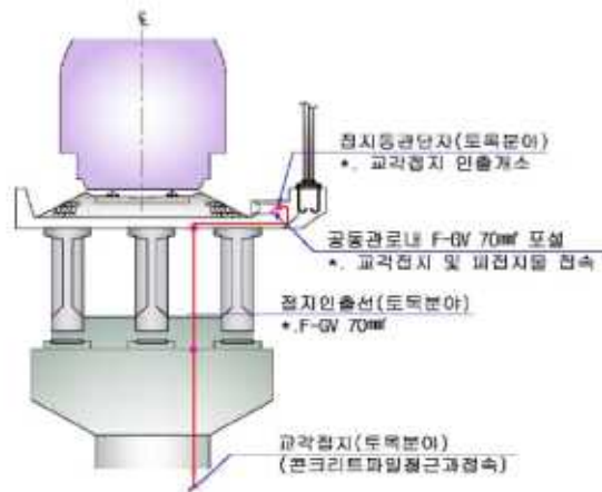
그림 36. 교량구간 접지설계 예(단선)
