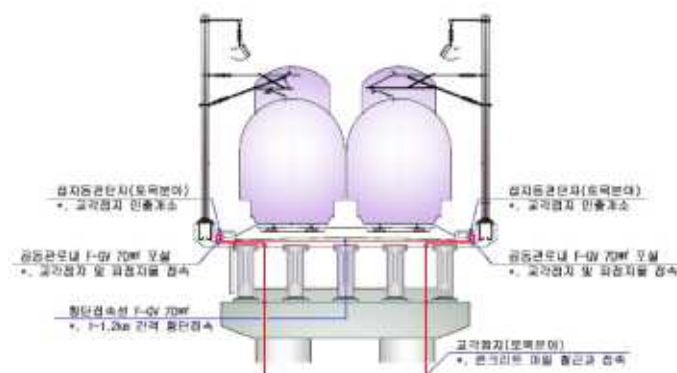
그림 35. 교량구간 접지설계 예(복선)
