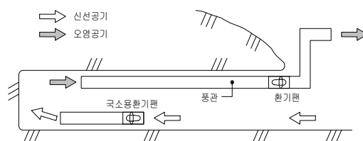
그림 40. 집중 배기식(덕트 내 부압)
