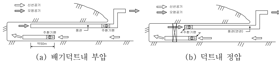
그림 48. 집중 급배기 조합식
