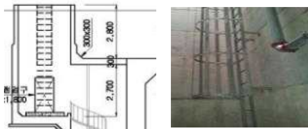
그림 21. 고정식 안전사다리 설계 예
