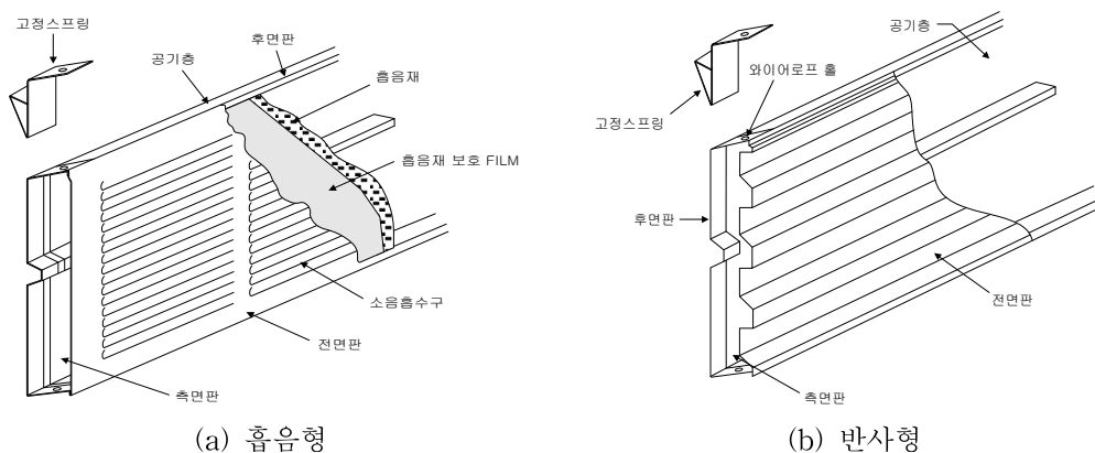
그림 5. 방음벽의 기본 구조형상
