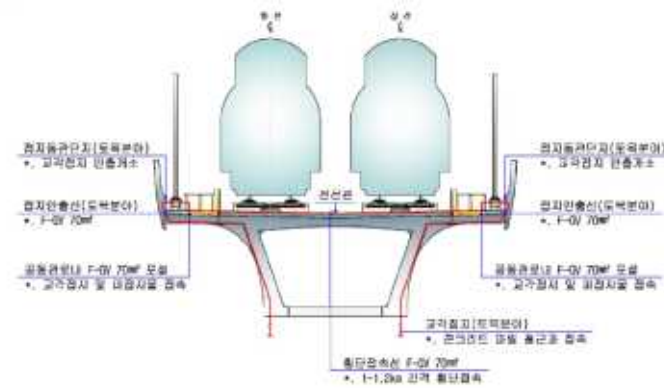
그림 29. 교량구간 접지설계 예
