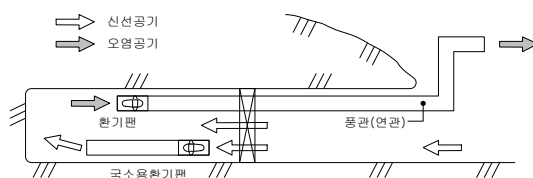
그림 41. 집중 배기식(덕트 내 정압)
