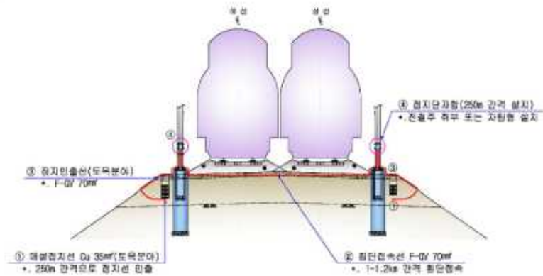
그림 31. 홑쌍기구간 접지설계 예(복선)
