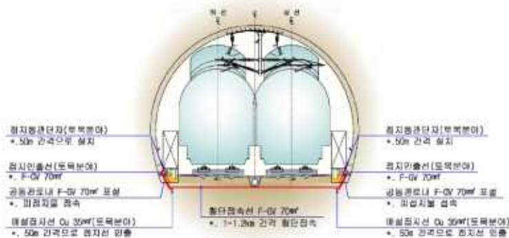
그림 30. 터널구간 접지설계 예
