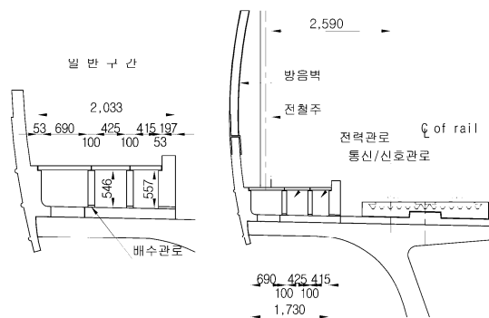
그림 26. 교량용 관로 설계 예
