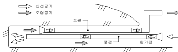
그림 47. 직렬 급배기 병용식
