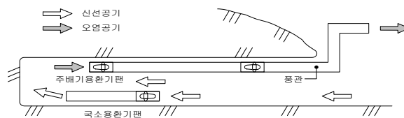
그림 43. 직렬 배기식(덕트 내 정압)
