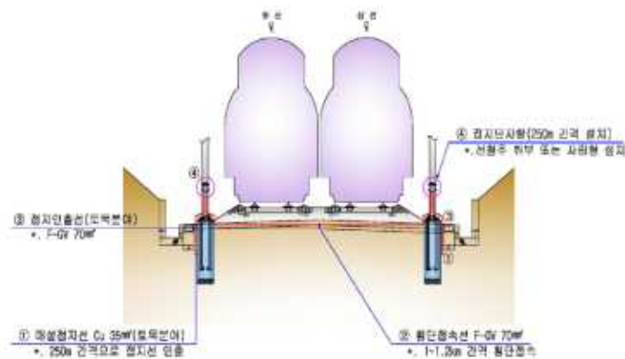
그림 32. 짝기구간 접지설계 예(복선)
