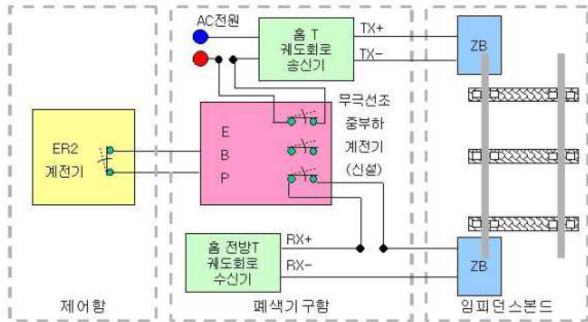
그림 19. 무연동의 인터페이스
