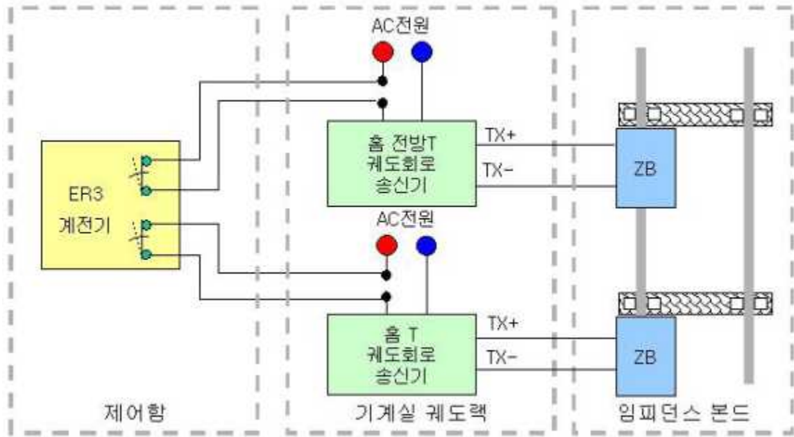
그림 18. 연동역 인터페이스
