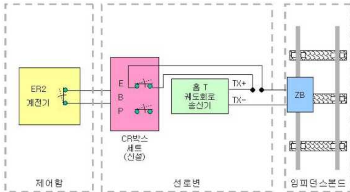
그림 21. 차내신호구간 인터페이스(무연동역)
