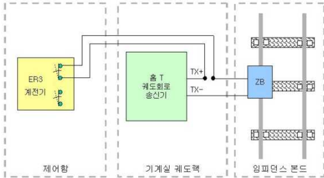
그림 20. 차내신호구간 인터페이스(연동역)
