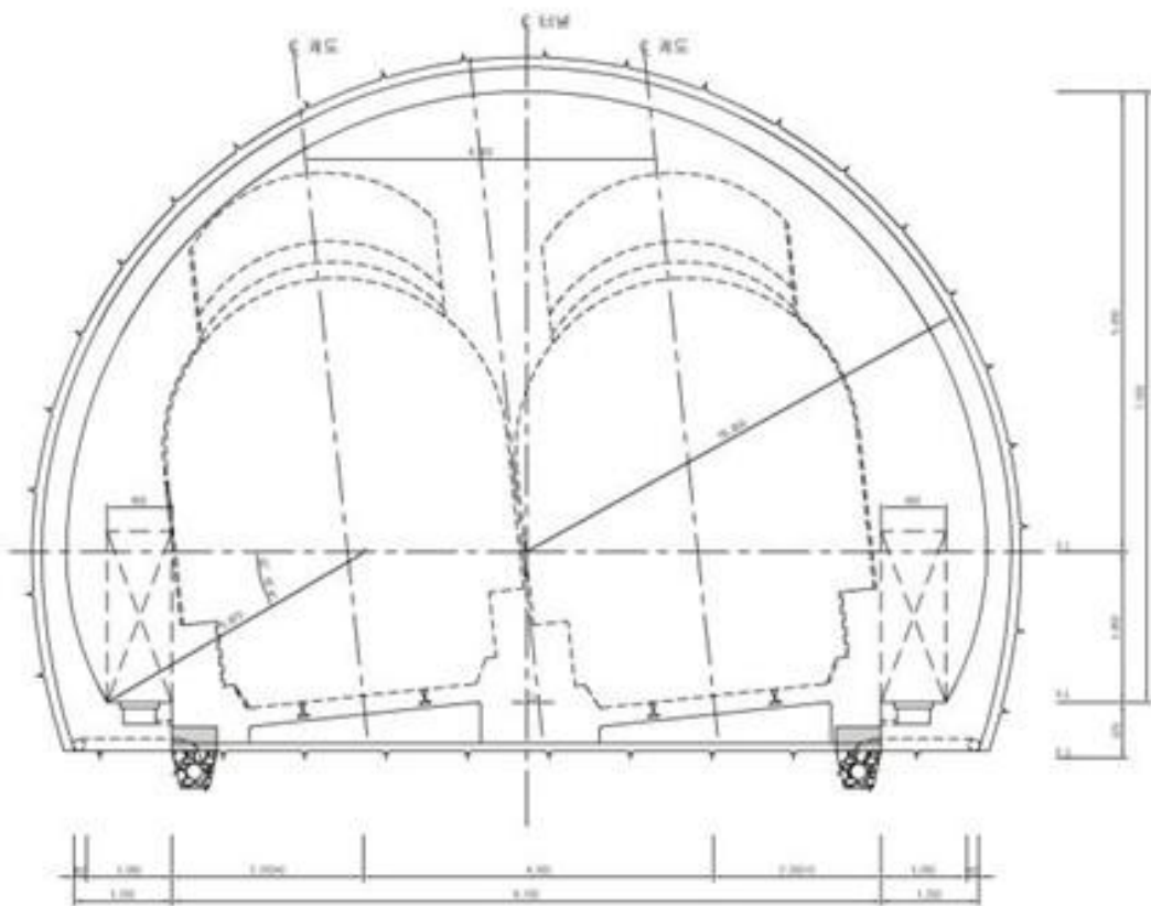
라. 선로중심간격 4.3m
