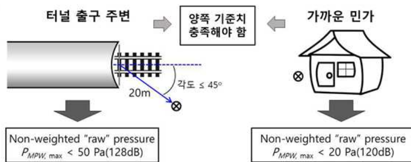
그림 3. 터널 미기압과 관리기준치
