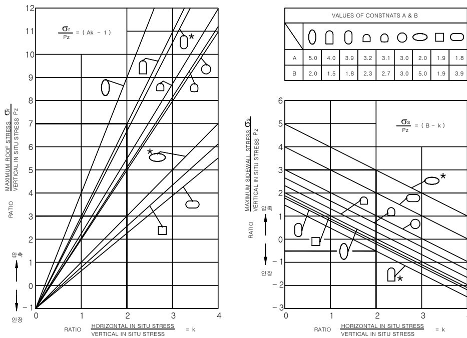
그림 17. 터널형상과 측압계수의 상관성에 따른 터널주변의 응력집중
