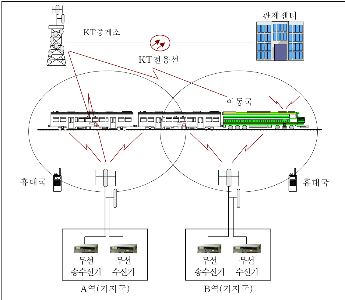
그림 1. 중계방식 구성도
