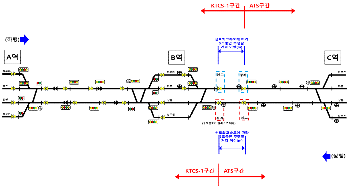
그림 2 ATS ↔ KTCS-1운전모드 변경 구간의 일반적인 구성도
