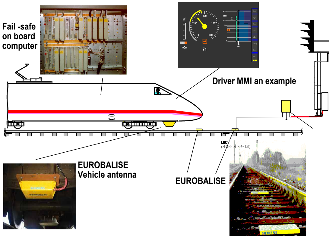
그림 7. 유럽열차제어시스템 구성
