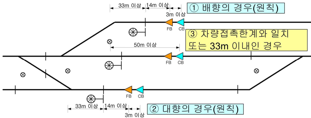
그림 1. 역구내 출발신호기 발리스 설치
