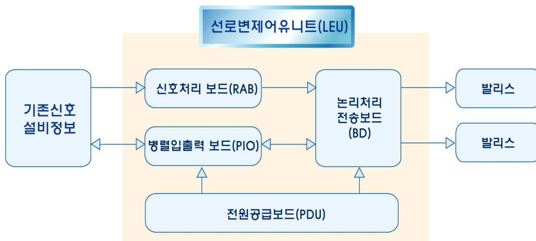
그림 20. LEU 구성도
