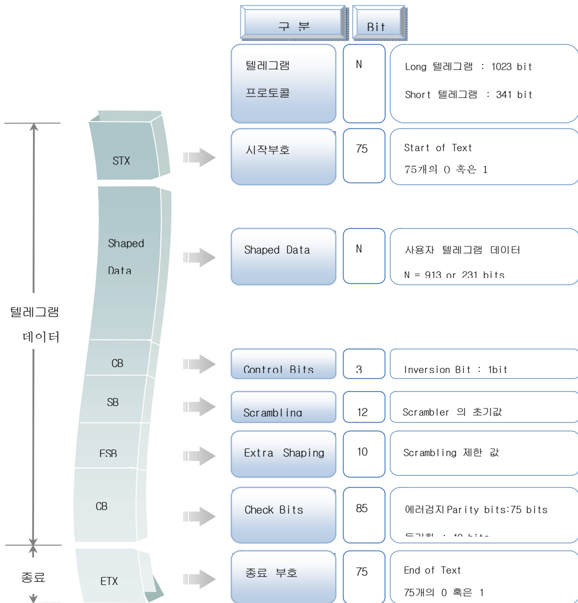
그림 29. 텔레그램 형식
