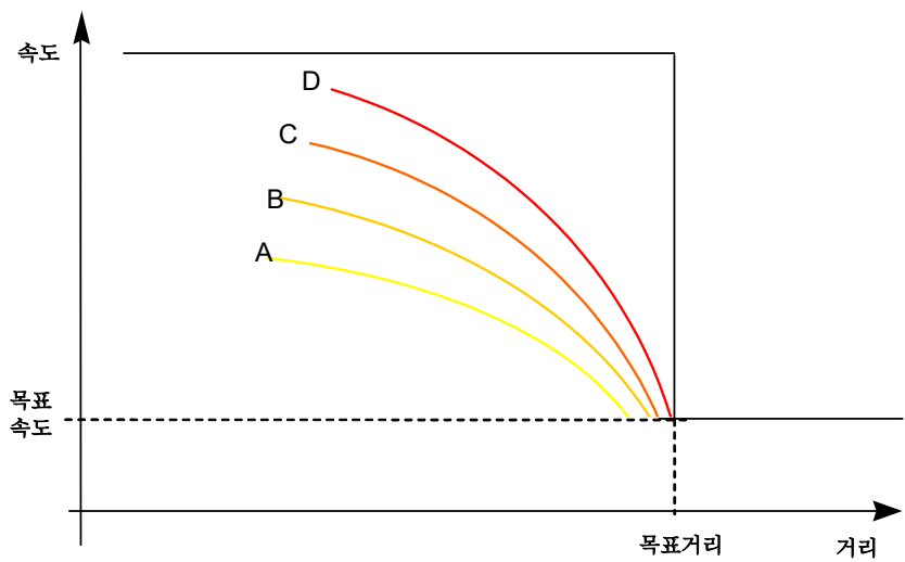
그림 13. 속도곡선
