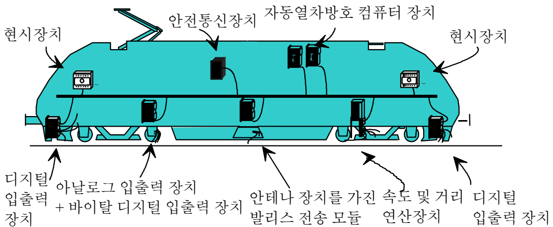
그림 9. 차내시스템의 분산설치(예)
