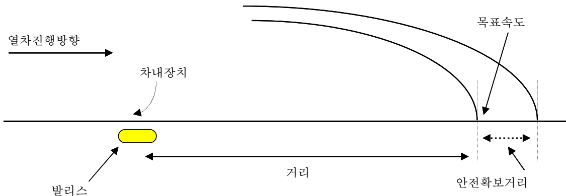
그림 10. 기본 제동곡선
