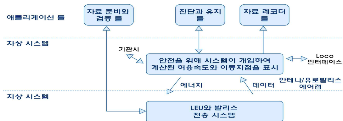
그림 15. ERTMS/ETCS시스템의 구조
