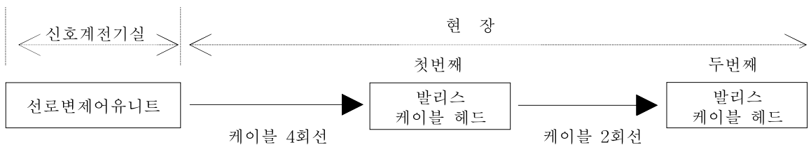
그림 3. 선로변제어유닛과 발리스 단자함간 케이블 설치도
