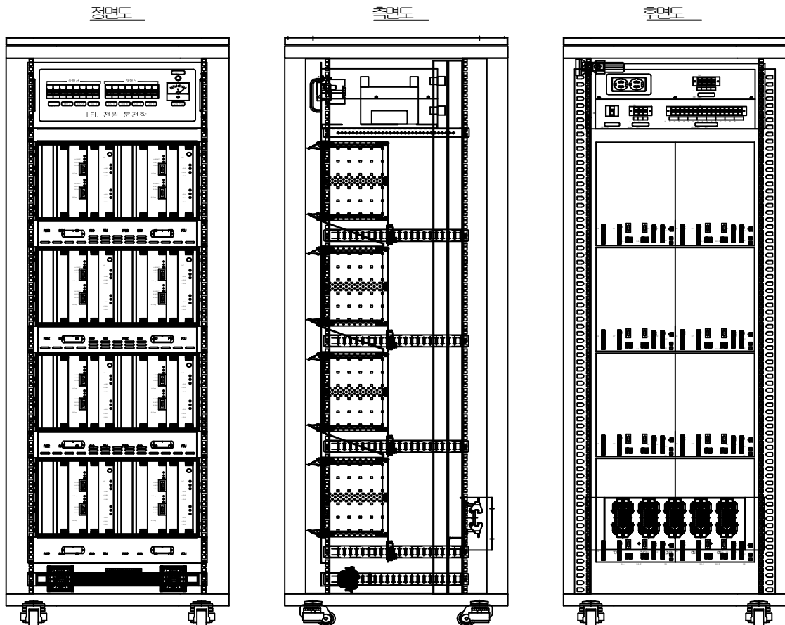
그림 18. 선로변제어유니트(실내용)(신호계전기실) 구성(LEU 서브랙 8개 기준)
