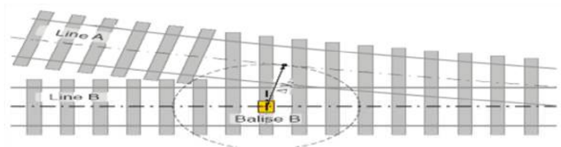
그림 26. 분기기 내의 발리스와 안테나의 최소거리
