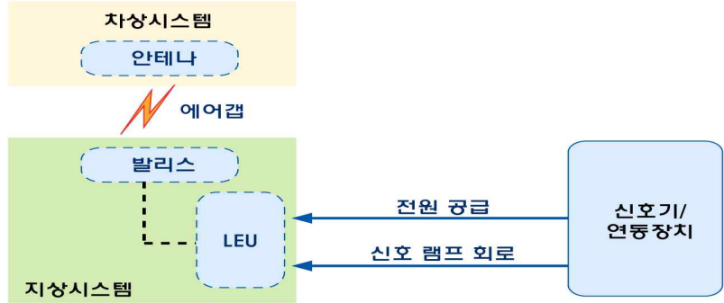
그림 16. 지상시스템 구조
