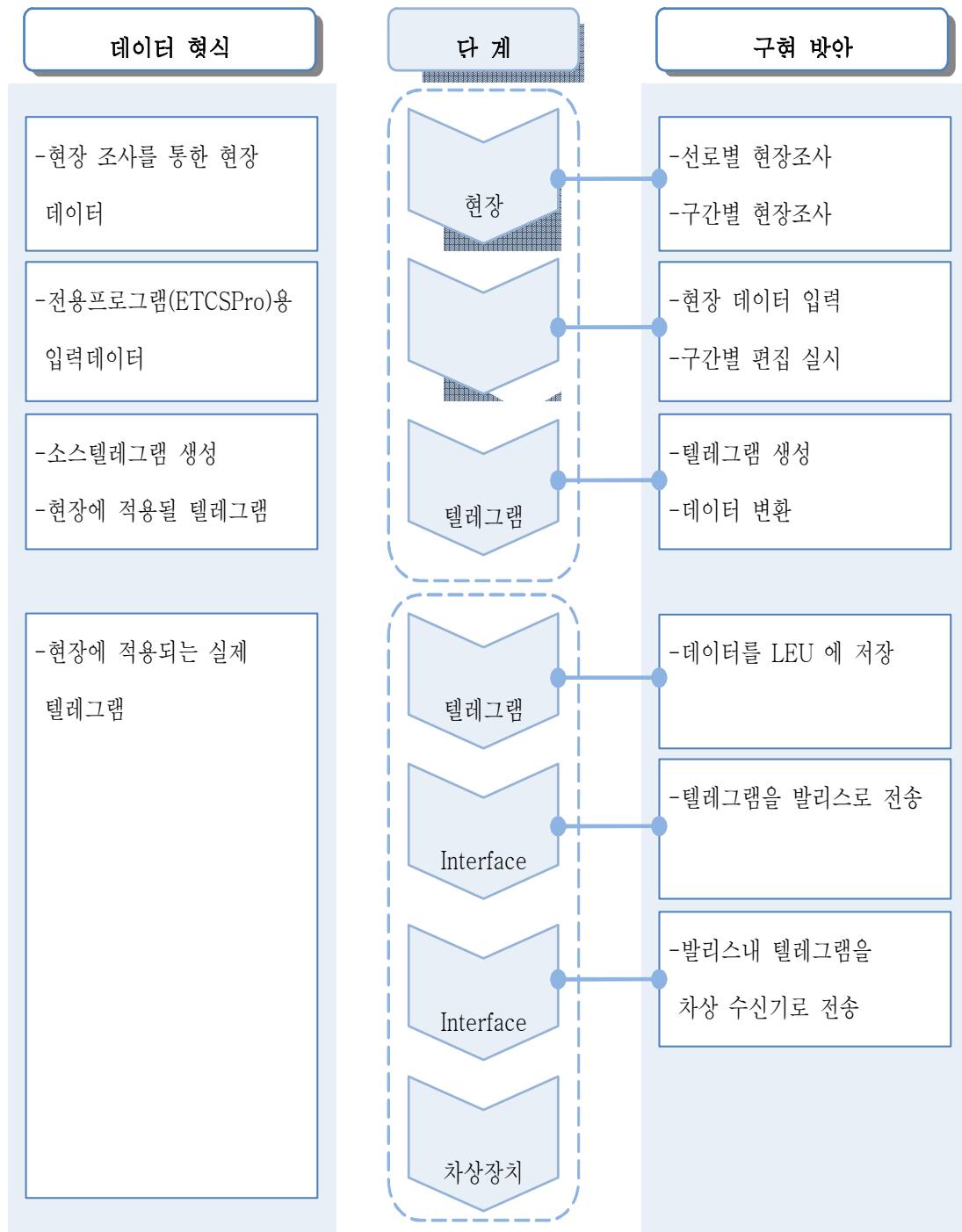
그림 28. 텔레그램 생성
