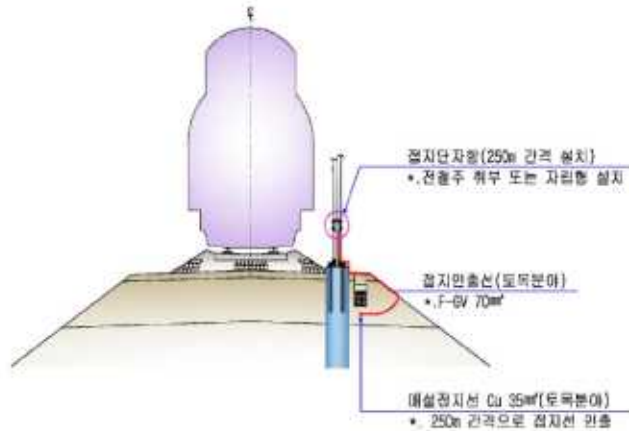
그림 32. 흙쌓기구간 접지설계 예(단선)
