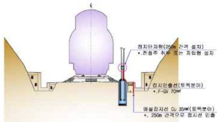
그림 33. 깎기구간 접지설계 예(단선)
