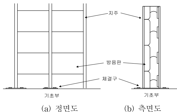
그림 5. 방음벽의 기본 구조형상
