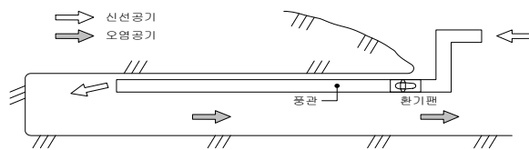
그림 43. 집중 급기식 환기개요도
