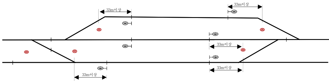
그림 4. KTCS-1 및 ATS/KTCS-1 혼용구간의 경우
