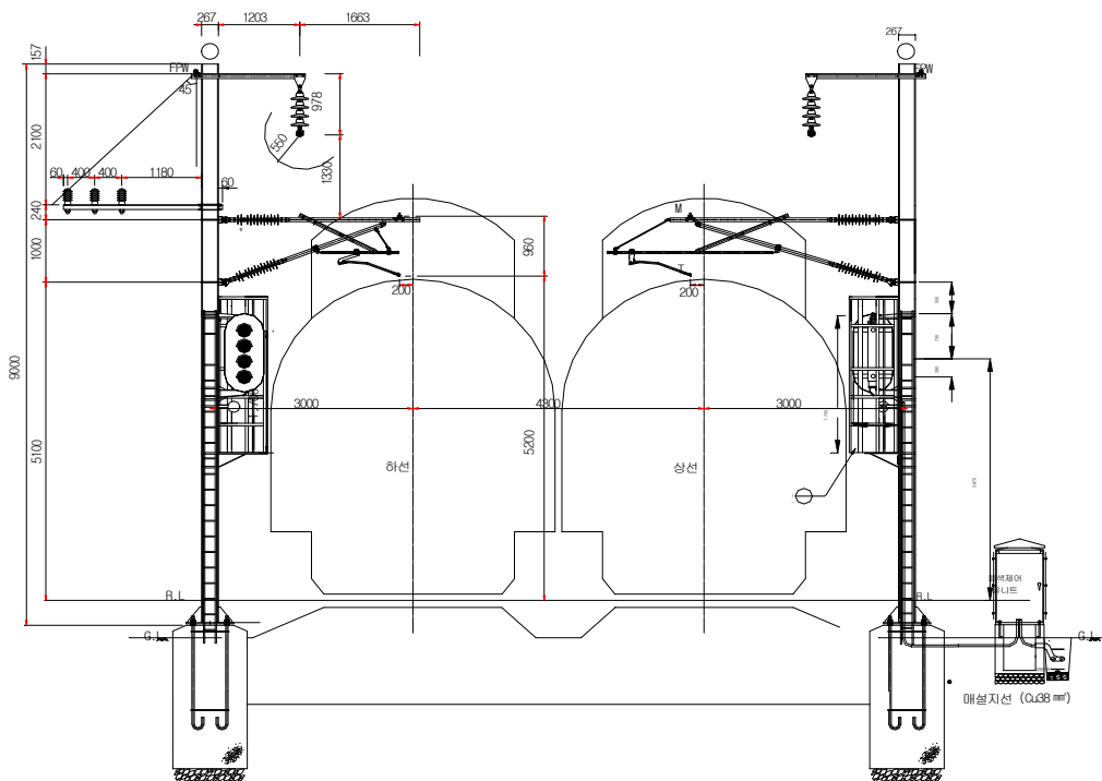
그림 30. 전철주에 신호기 설치[mm]
