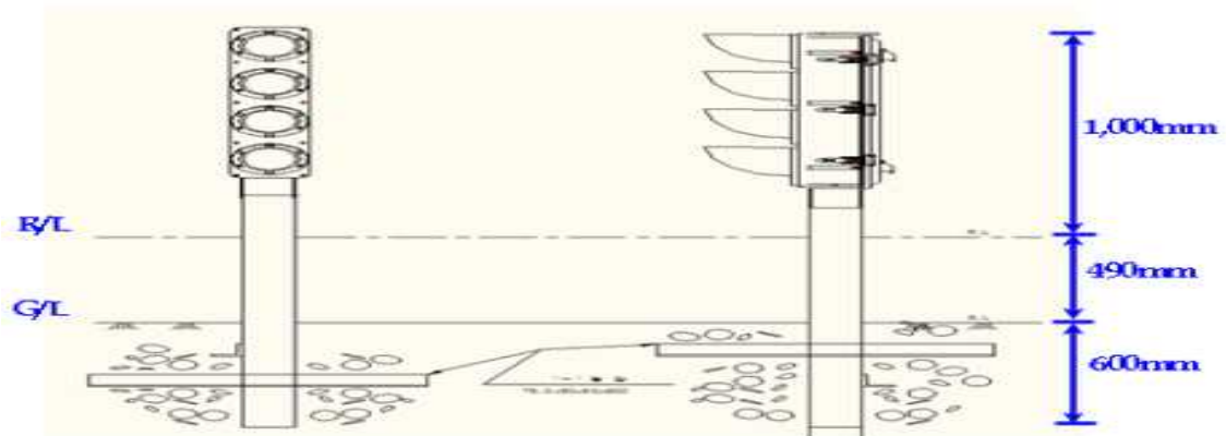
그림 35. 보조신호기 설치
