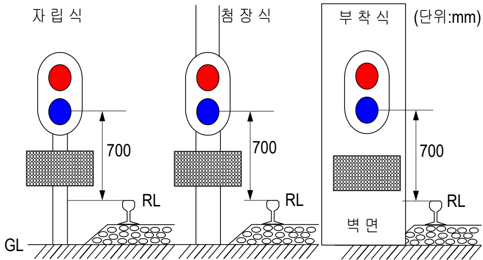
그림 13. 입환표지
