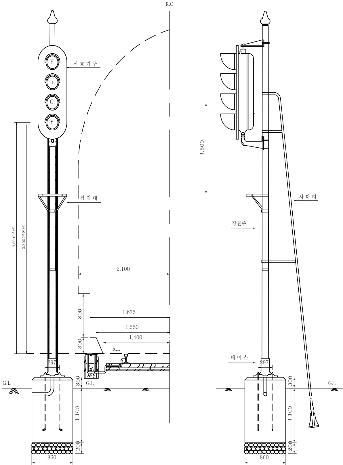
그림 27. 토공구간 신호기 설치[mm]
