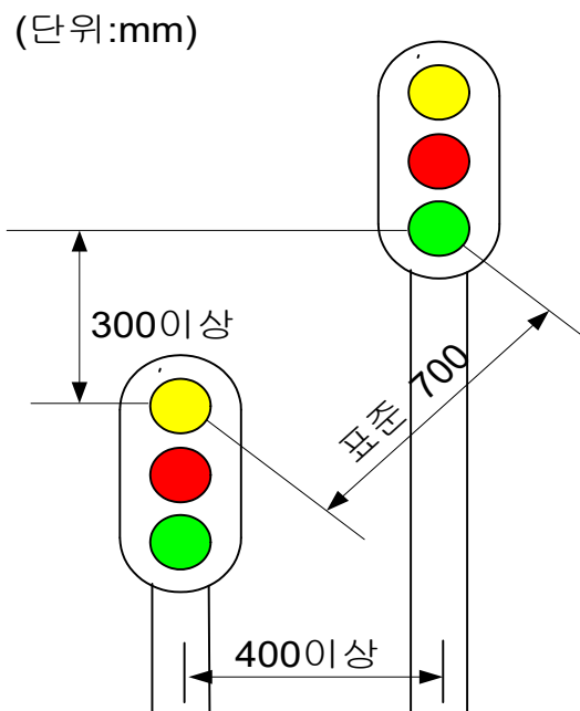
그림 15. 출발신호기간 간격
