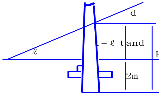
그림 31. 콘크리트 주의 모멘트
