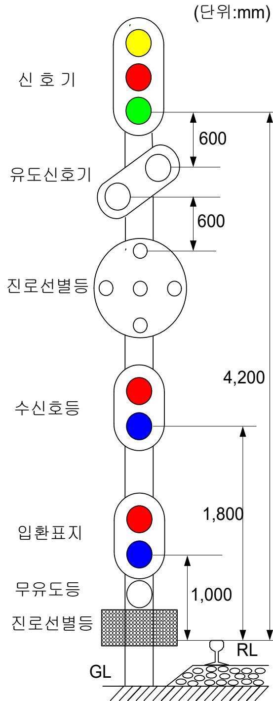
그림 19. 1주 다등의 경우 신호기간 간격
