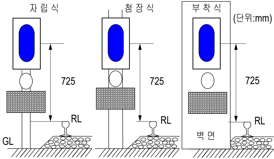
그림 10. 입환신호기
