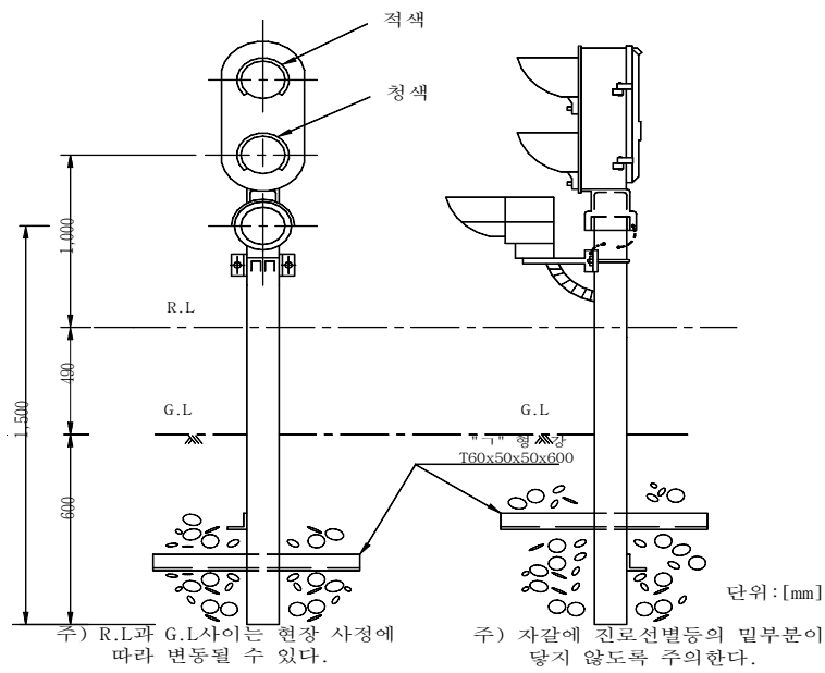
그림 32. 토공구간 입환신호기 설치[mm]
