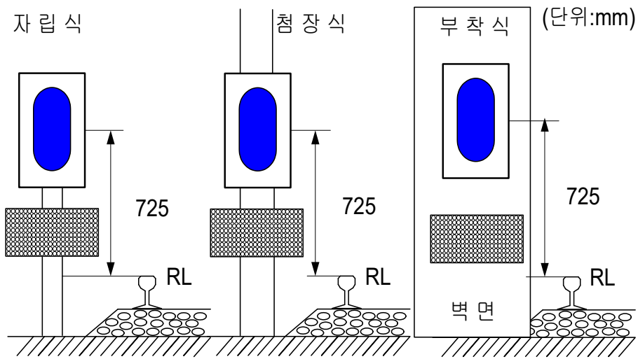
그림 11. 입환표지
