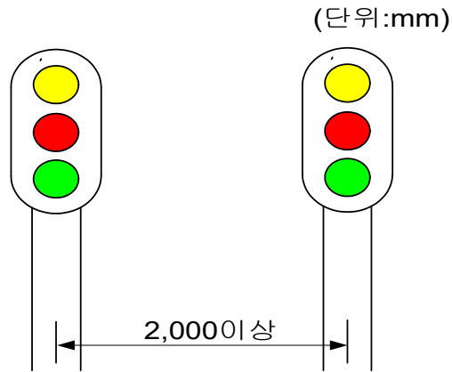
그림 16. 장내신호기간 간격
