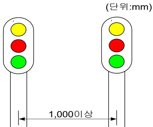
그림 17. 출발신호기간 간격
