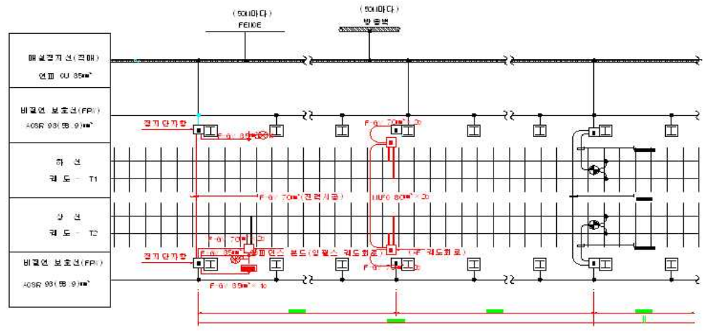
그림 3. 통합접지 계획도
