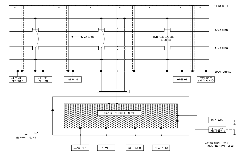
그림 2. 통합접지방식의 구성도
